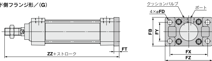
ヘッド側フランジ形
