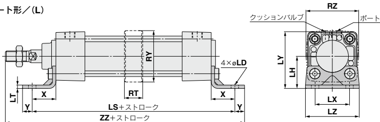
フート形 (mm)
