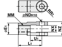
Y形二山 ナックルジョイント
