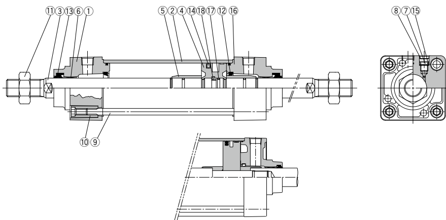
MBW125の場合
