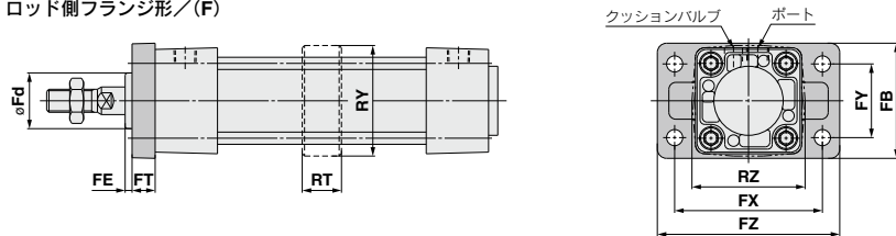
ロッド側フランジ形
